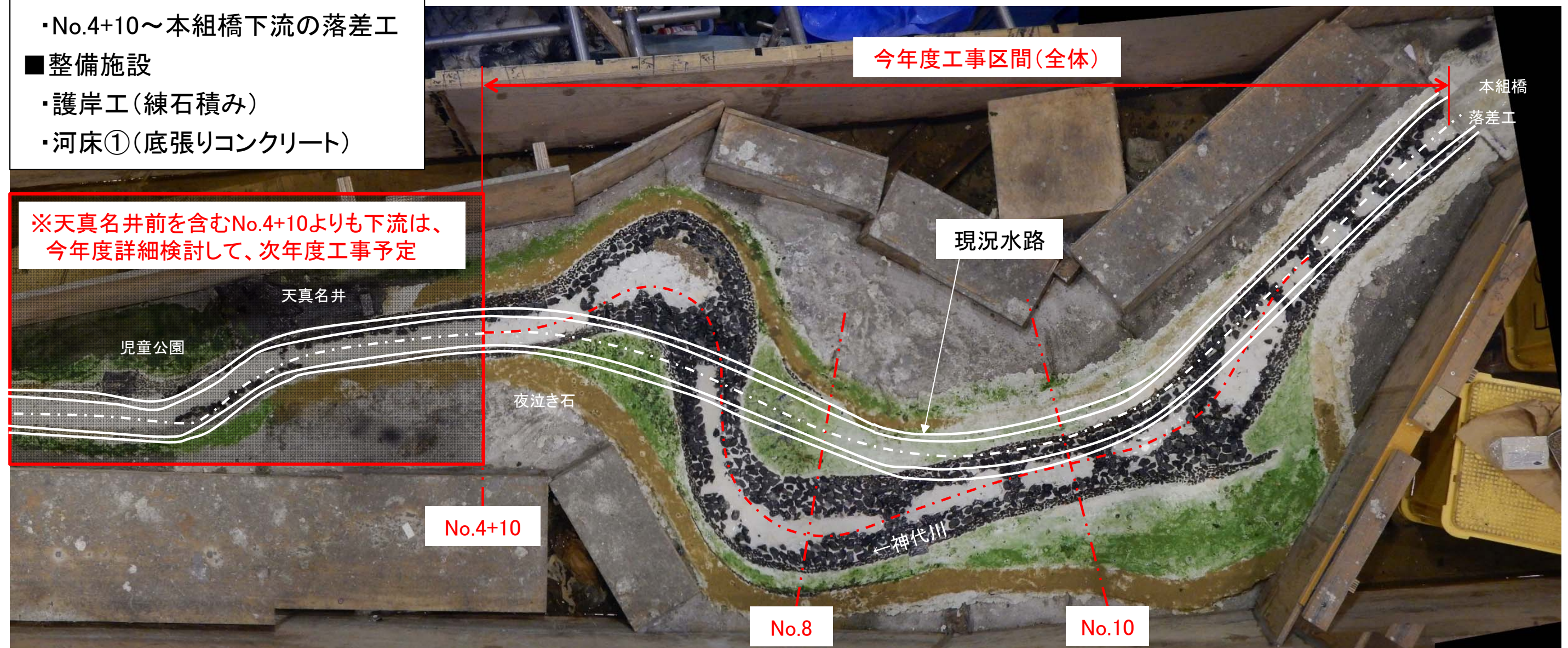
平面図
