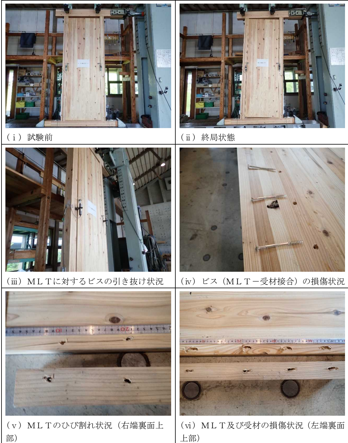
写真 2 出隅対応型－2 試験体の破壊性状
