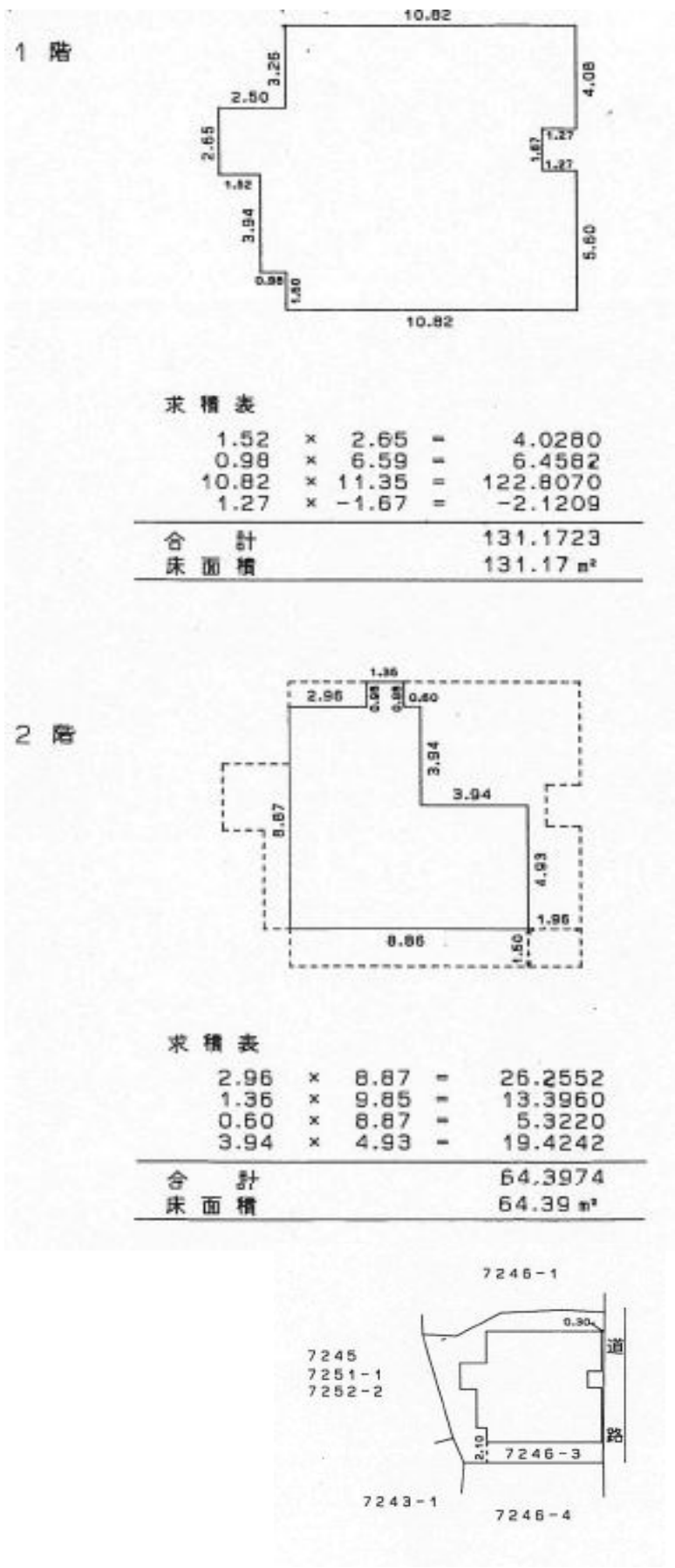
3) 求積図
