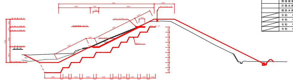
洪水吐工断面图 S=1:400
