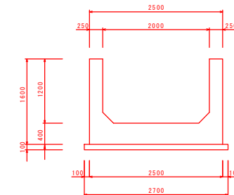
取水工断面図 501-400
