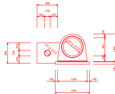
底樋断面図 S=1:100
