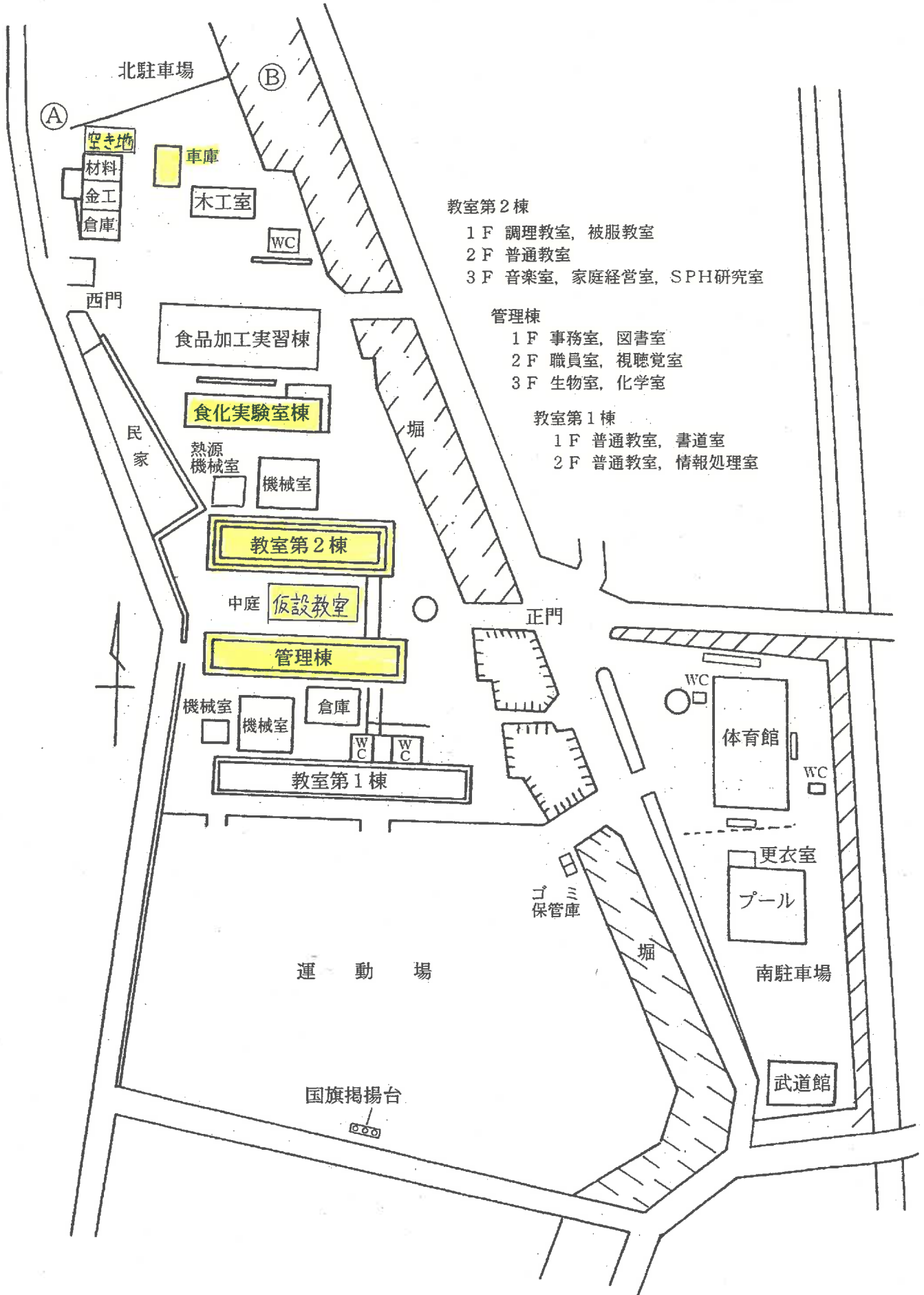
学校校舎配置図
