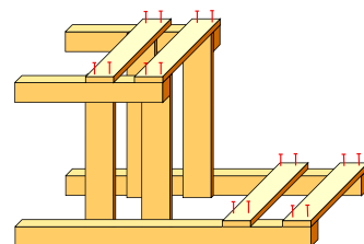
図 3 脚とまく板・背板の接合
