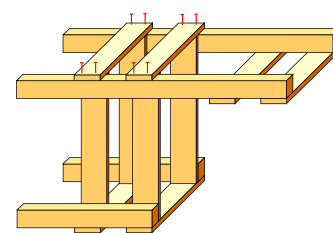
図 4 脚（長）とまく板の接合
