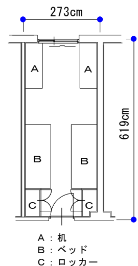
寮室平面図
