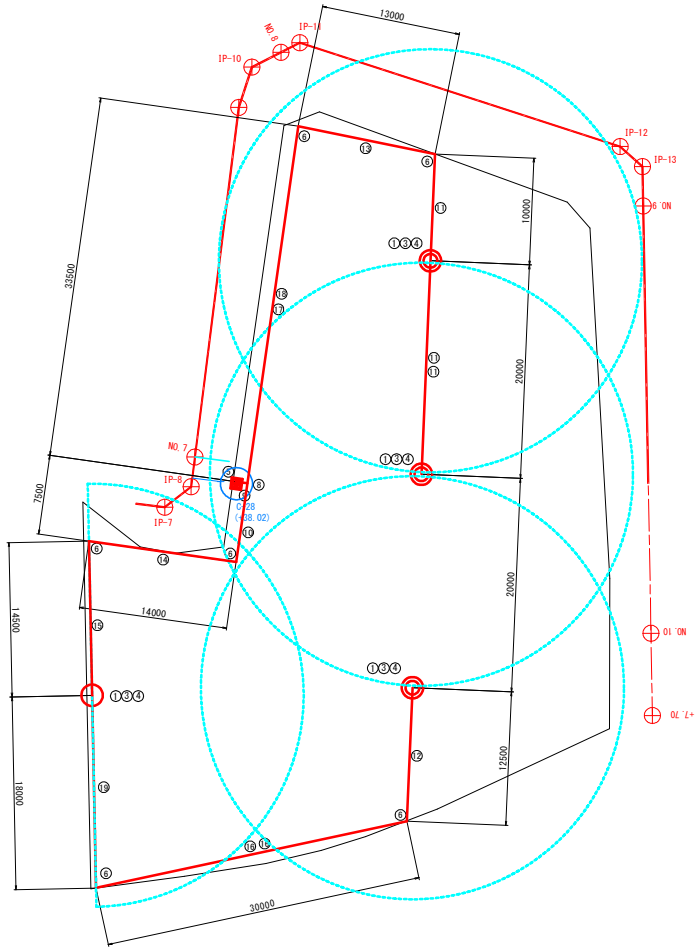
平面図 S-17-230
