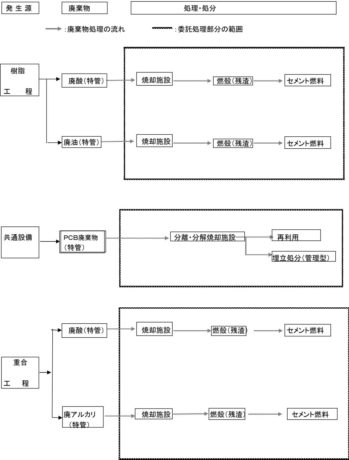
特管産業廃棄物処理フロー図（樹脂、重合、延プラ、共通）
