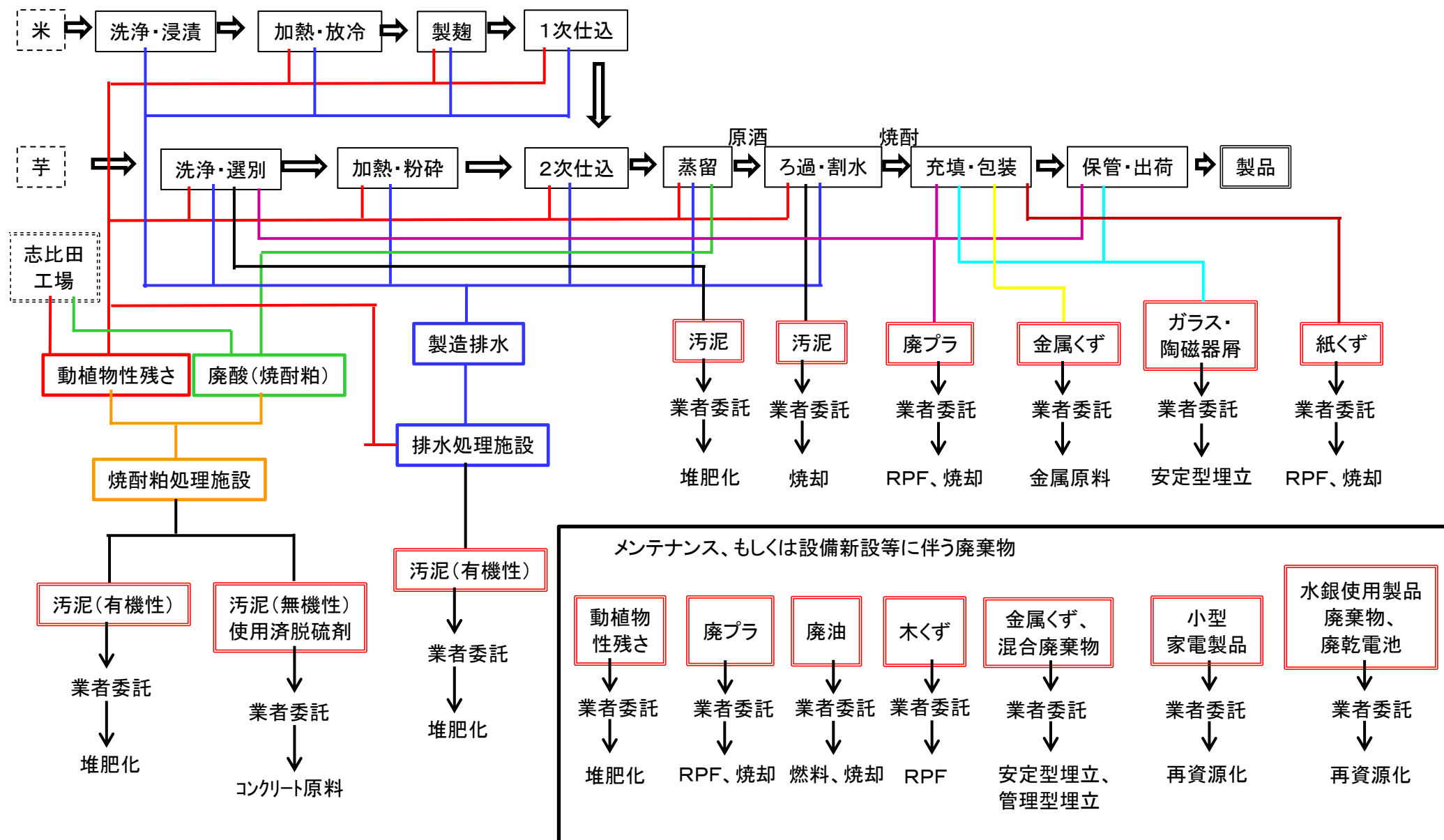
別添 図1 産業廃棄物の一連の処理工程(本社、本社増設工場)
