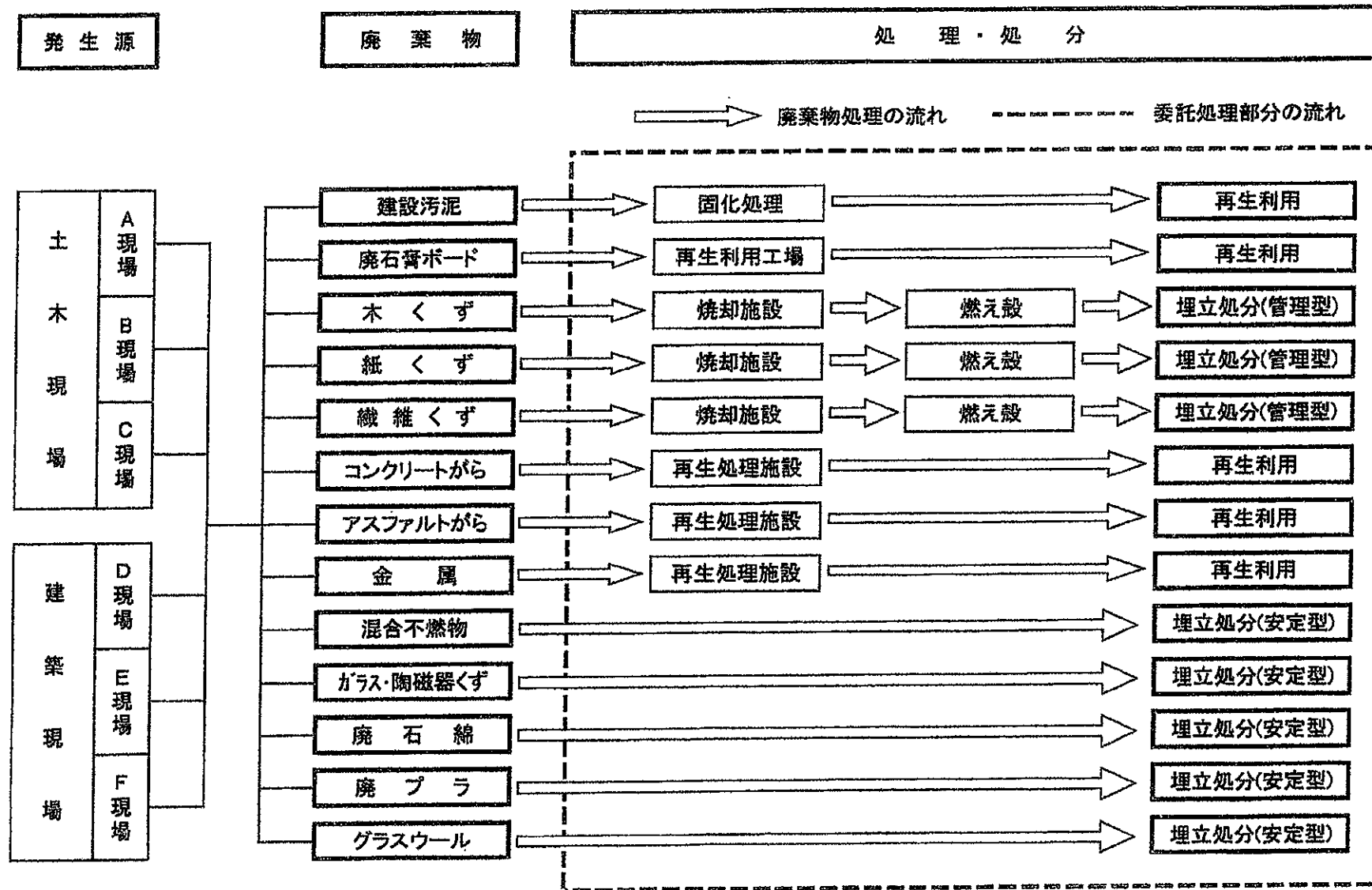
廃棄物処理フロー図(現状)
