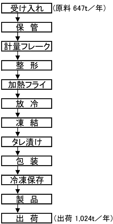
図4 惣菜工場フローシート (惣菜工場)
