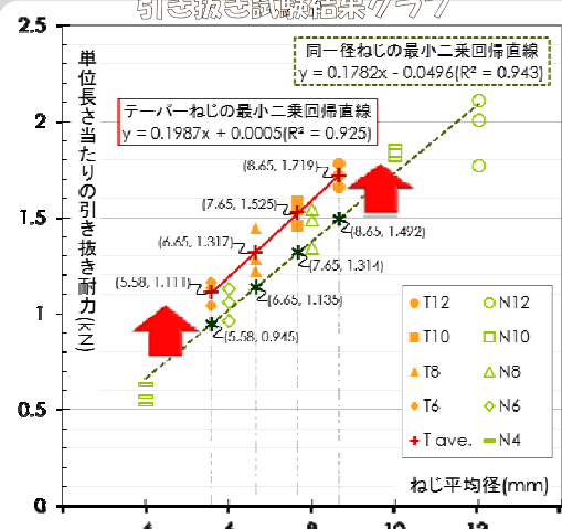
引き抜き試験結果グラフ
