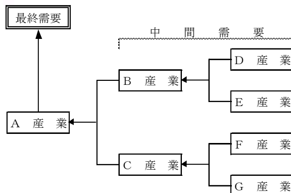
図3-4 需要と生産
