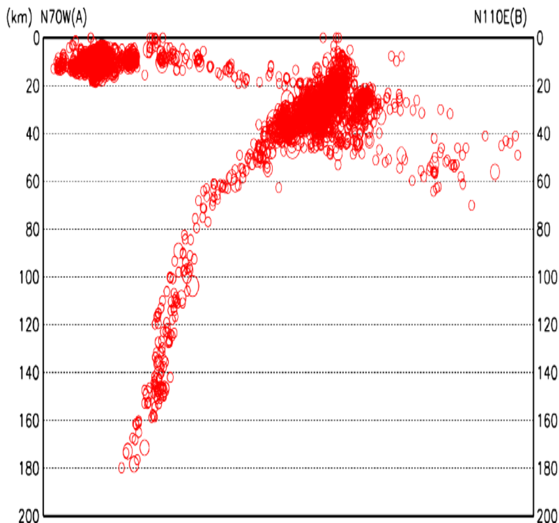
図 1-2 図 1-1 の破線 A—B からみた断面図
