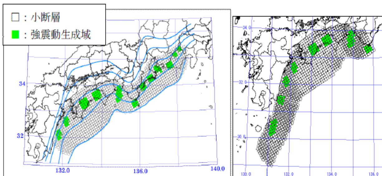
強震断層モデル （左）内閣府モデル（M9.0）
