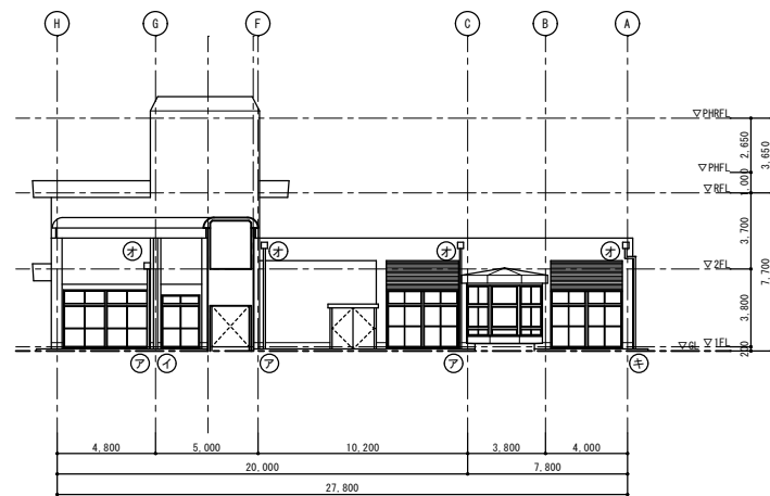
既存西立面图 S=1/200
