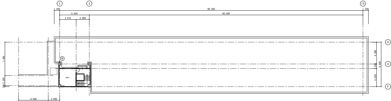
既存R階平面図 S=1/200
