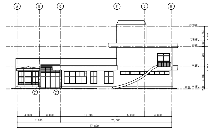
既存東立面図 S=1/200
