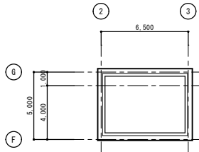
既存PH階平面図 S=1/200
