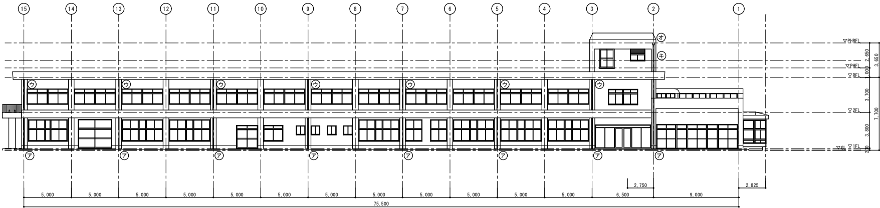
既存北立面図 S=1/200
