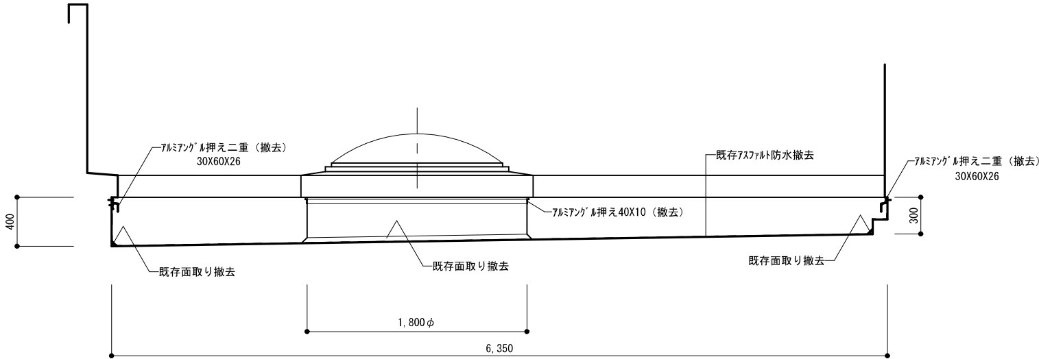
改修前 A 断面詳細図 S=1/30
