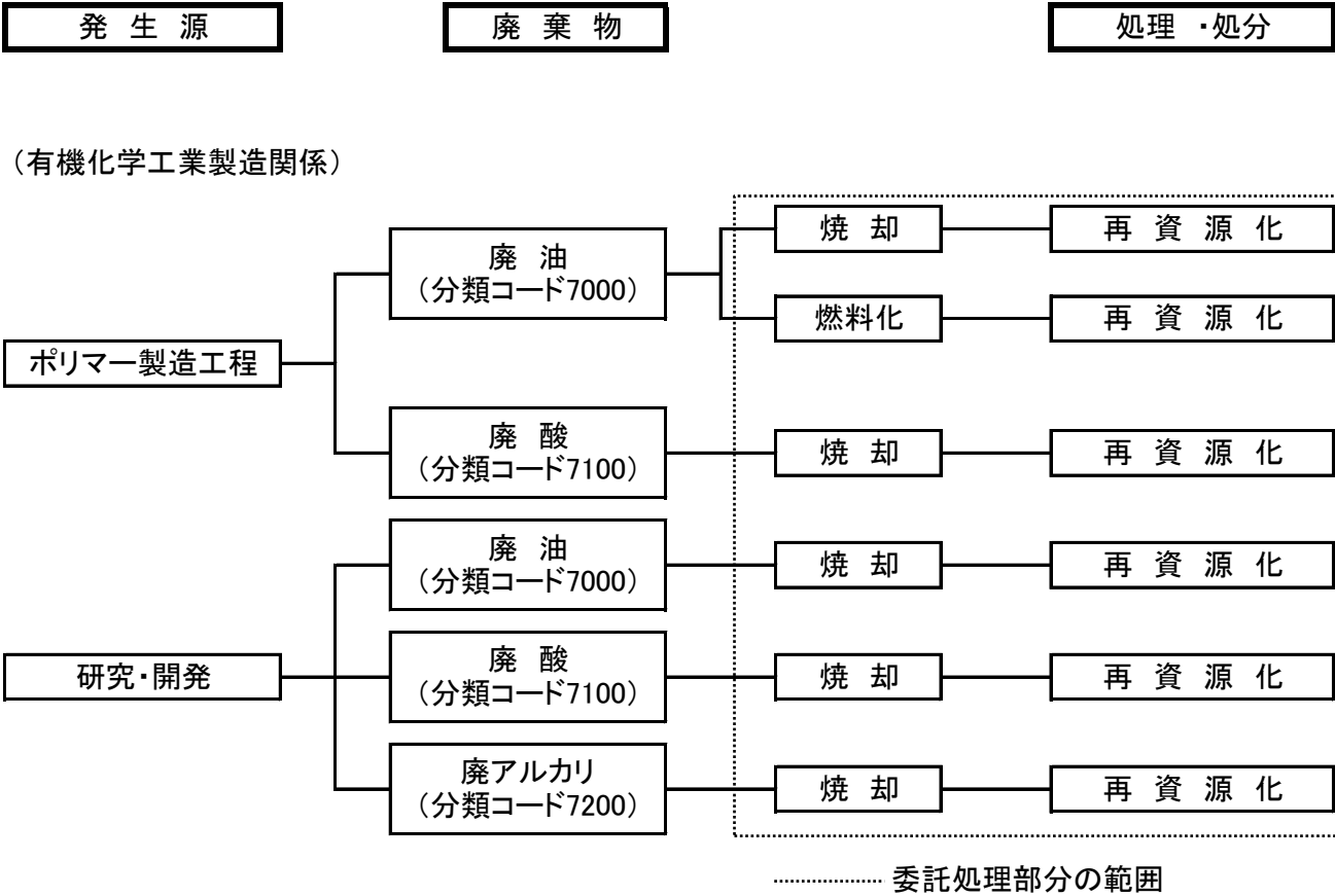
特別管理産業廃棄物処理フロー図
