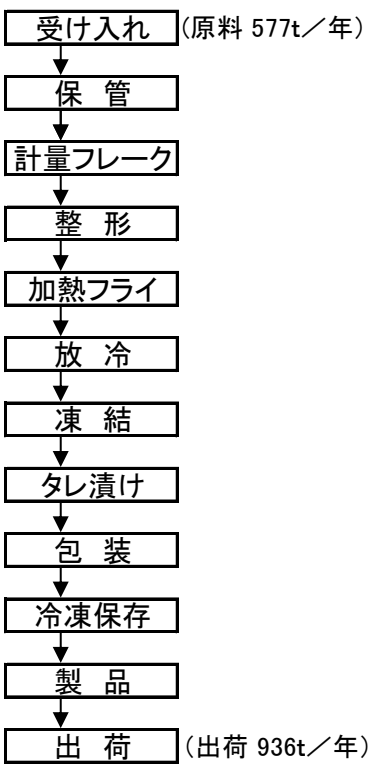
図4 惣菜工場フローシート (惣菜工場)
