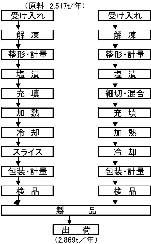
図1 ハム・ソーセージ製造フローシート (製造工場)
