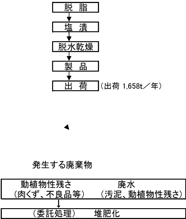
図5 原皮工程フローシート (原皮工場)
