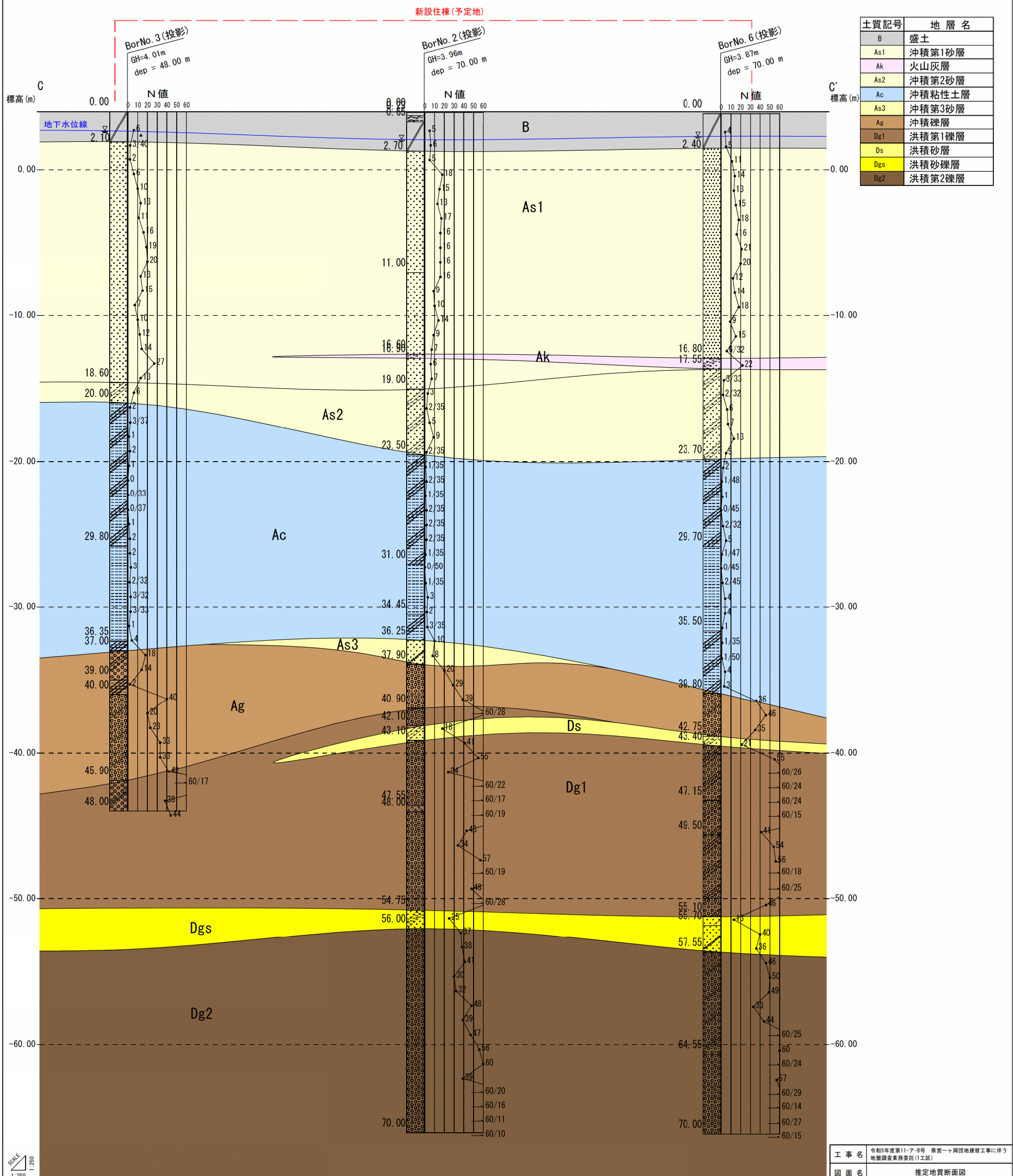
C-C' 推定地質断面図 縮尺A3(1:250)
