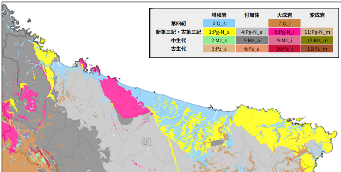
図-1.1.6 地質図
