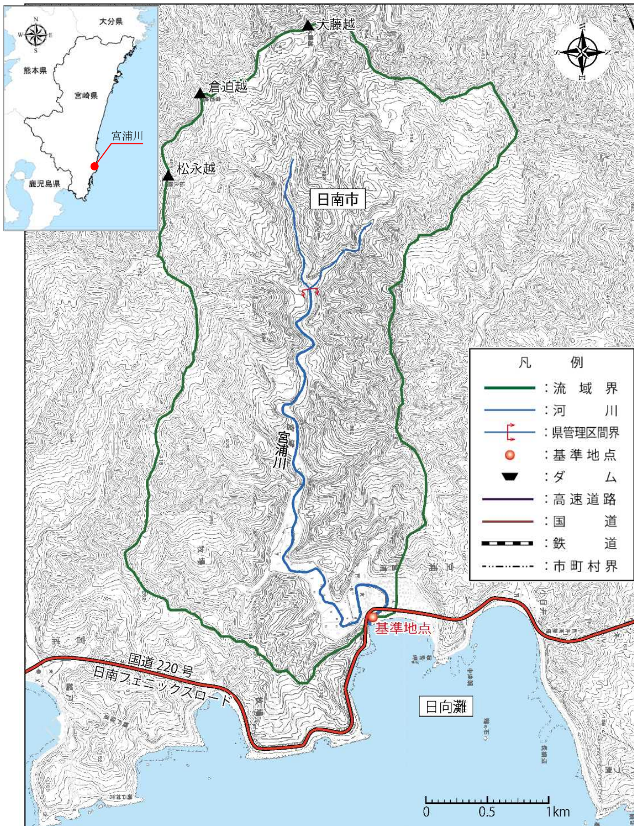
(参考図) 宮浦川水系図
