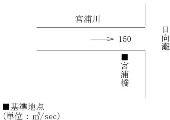
宮浦川計画高水流量図
