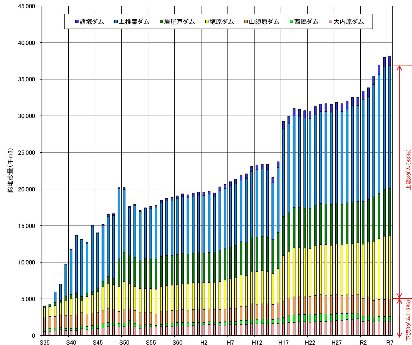
図1-6 ダム堆砂量の経年変化
