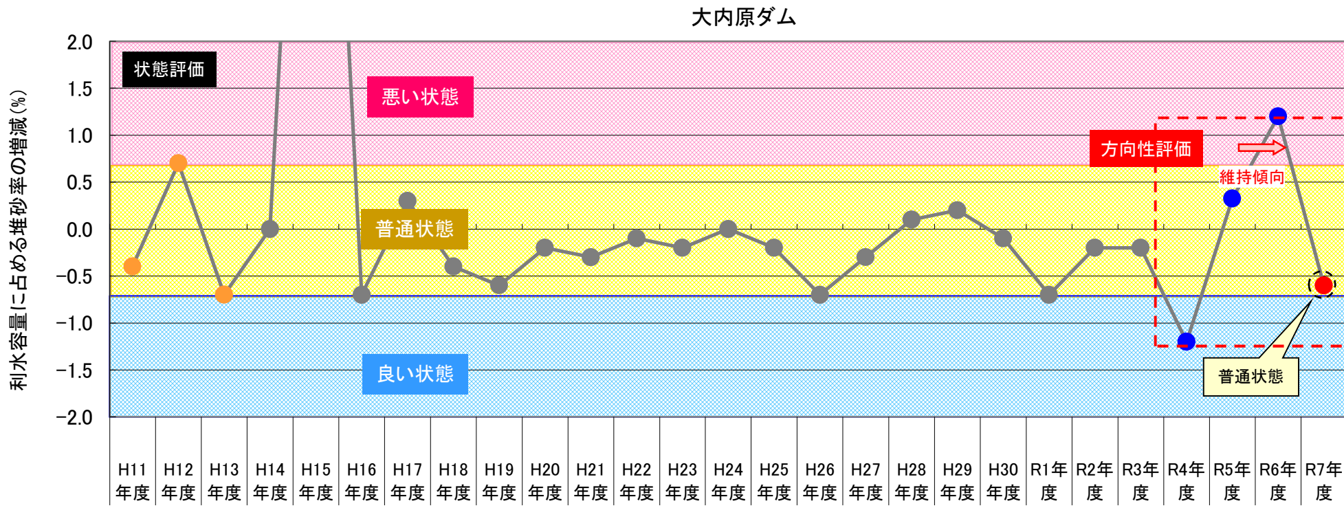
図10-2(3) 利水容量に占める堆砂率の増減の推移（西郷ダム、大内原ダム）
