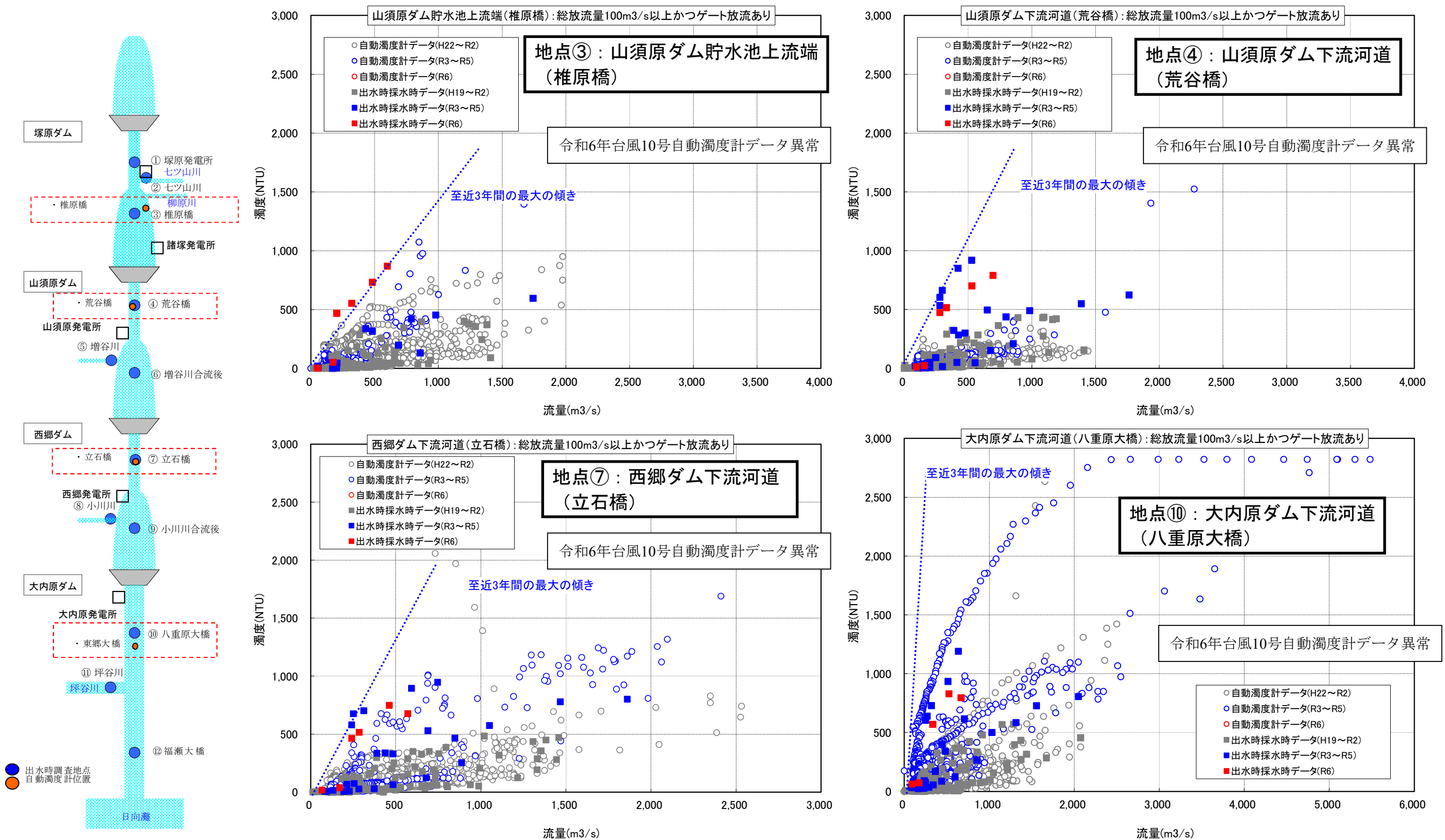
図14-3 流量規模別濁度の状況
