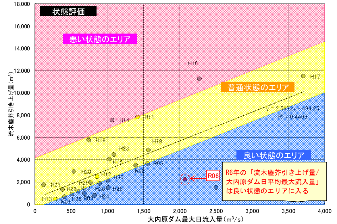
図12-3 流木塵芥引き上げ量と大内原ダム最大日流入量の相関図
