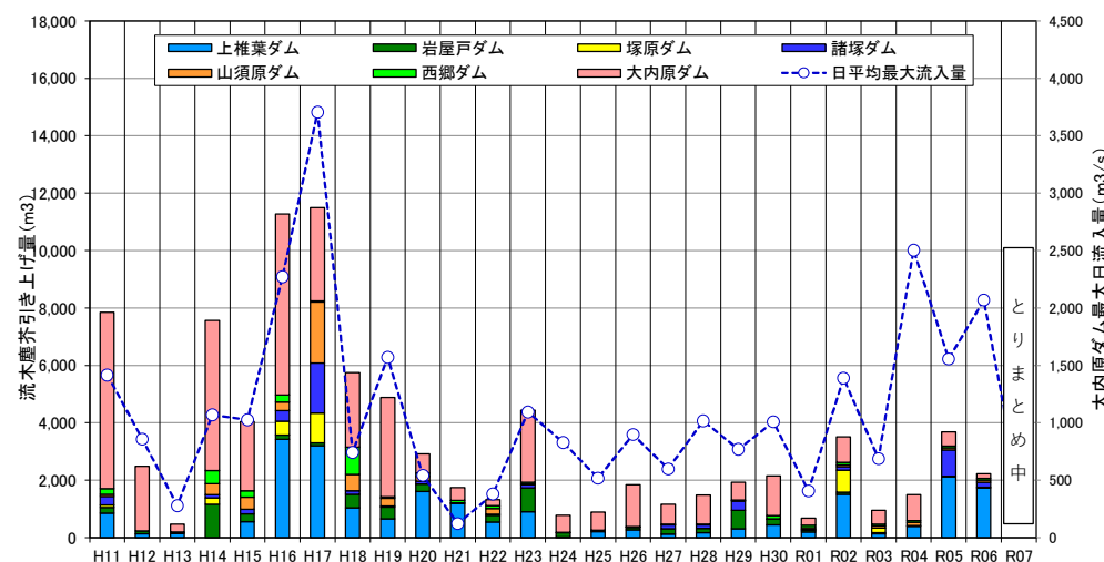
図12-1 流木塵芥引き上げ量と最大日流入量の推移
