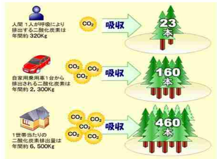
・身近な二酸化炭素排出量と森林（スギ人工林）の二酸化炭素吸収量
