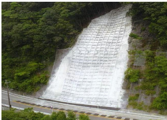
斜面補強（国道 327 号日向市船戸）
