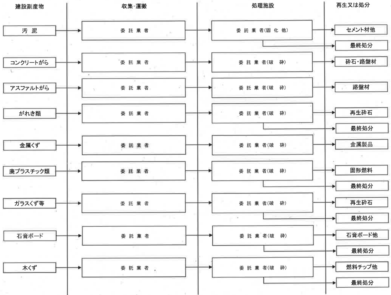
別紙1-1 産業廃棄物の一連の処理の工程
