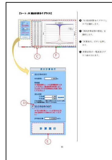
調整池計算システム
