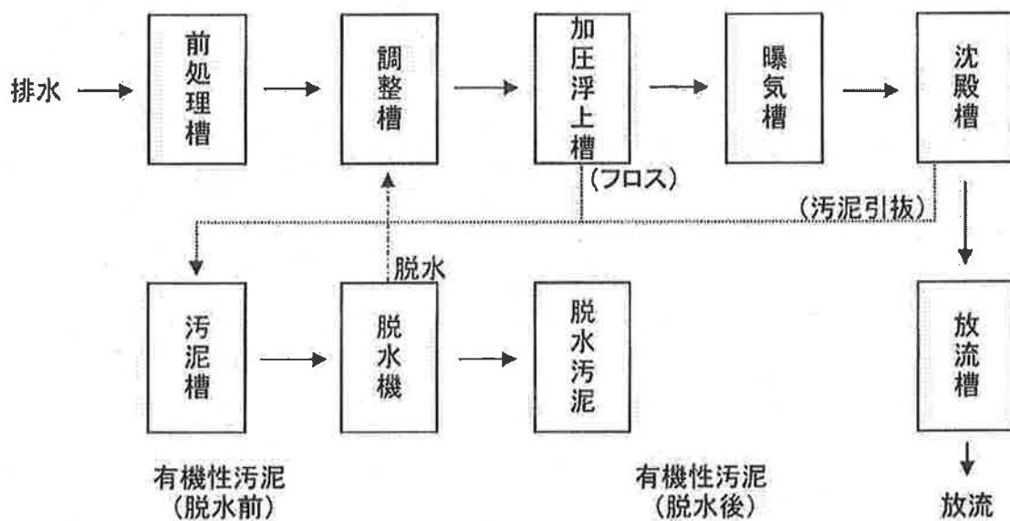
図2 排水処理フローシート
