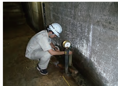
(漏水量測定)
