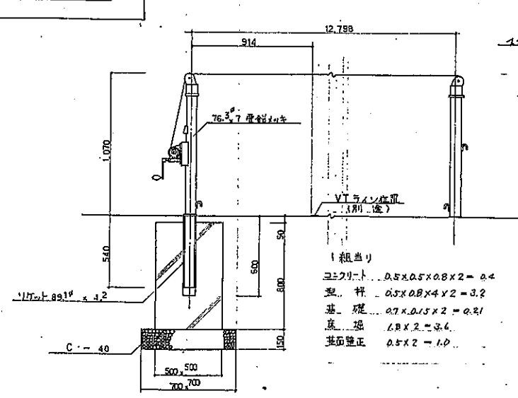
ネットポスト 詳細図 1/20
