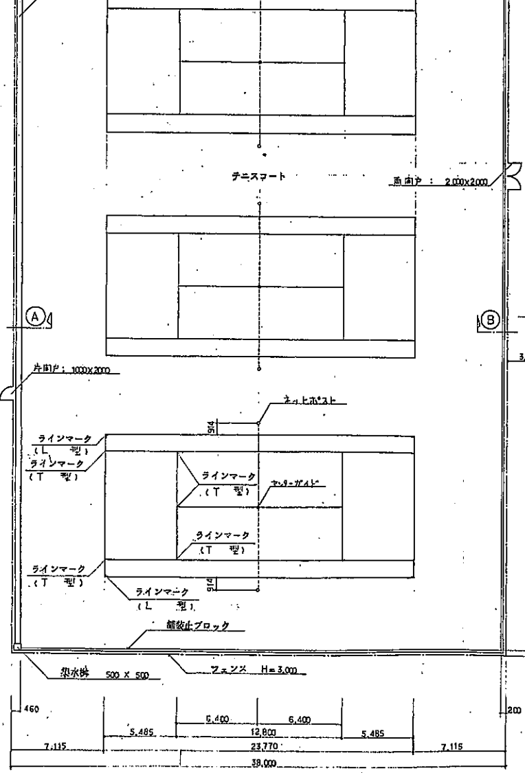
テニスコート ハンドボールコート 平面図 1/200
