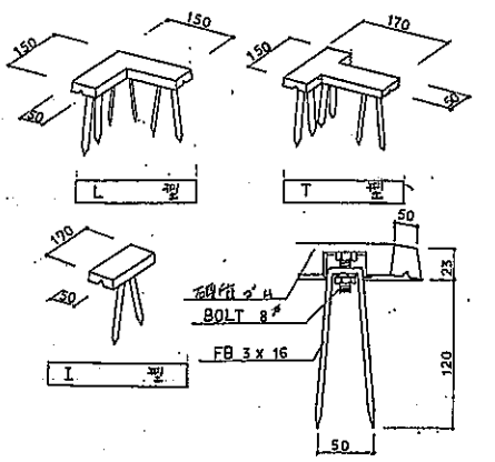
ラインマーク 詳細図
