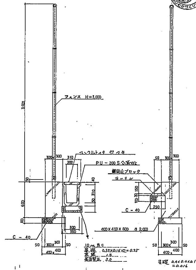
(A) 断面詳細図 1/20
