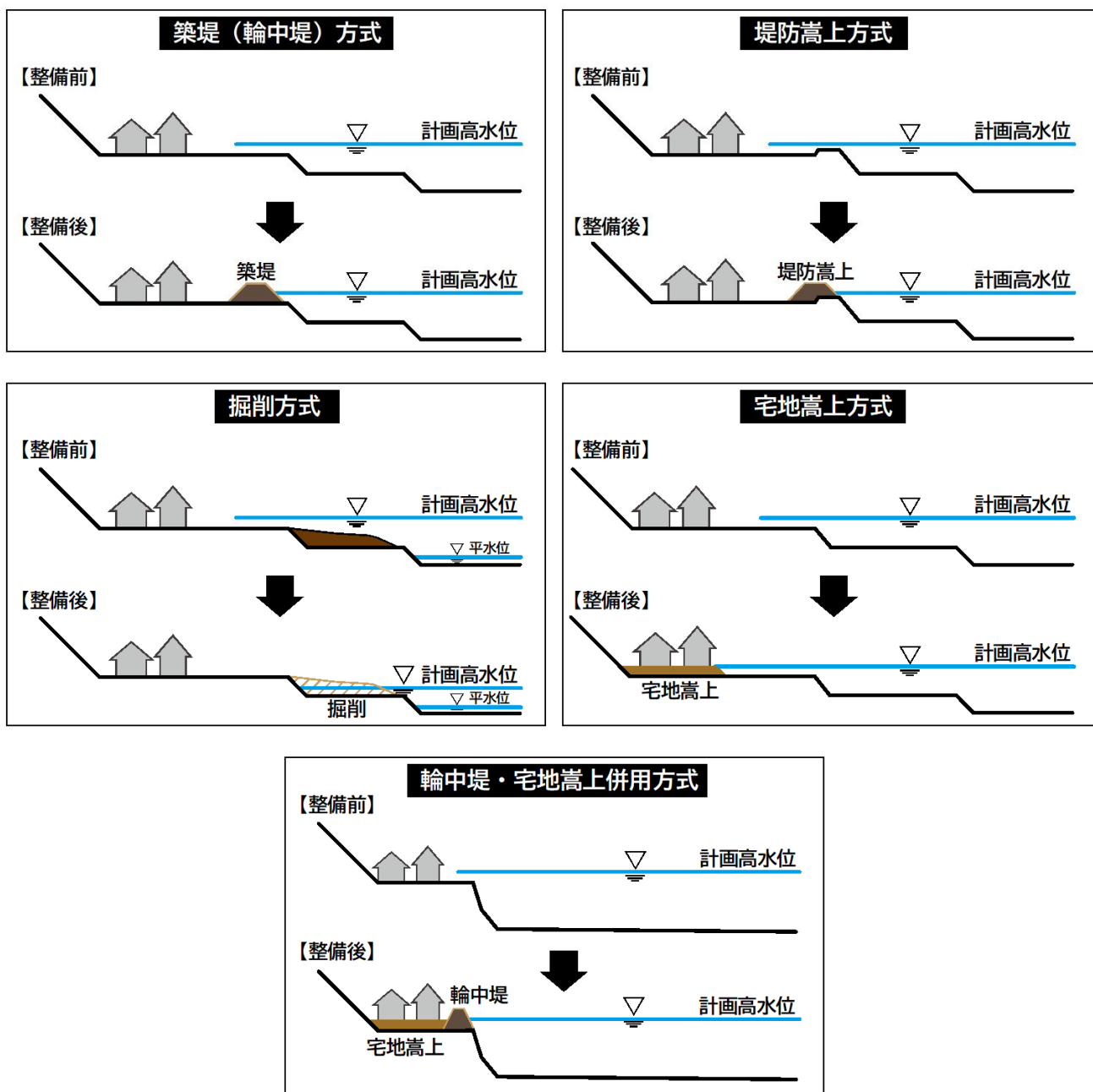
図一9 治水対策方式のイメージ図
