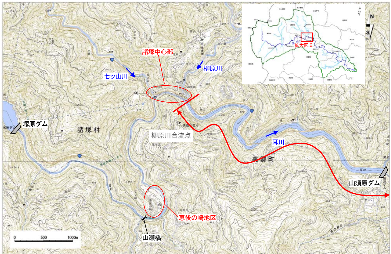
図-8 施行区間(拡大図、赤字:施行地区)
