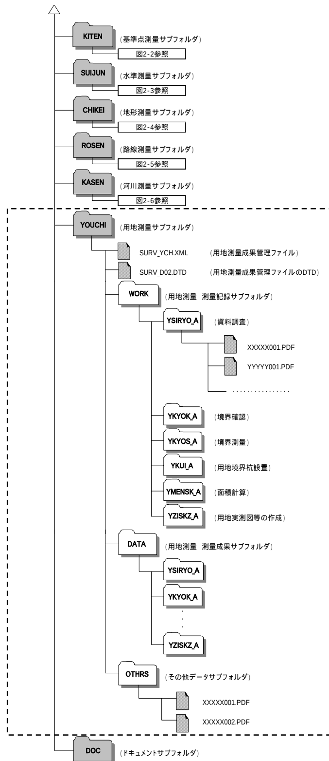
図 2-7 「YOUCHI」フォルダ内のサブフォルダ構成
