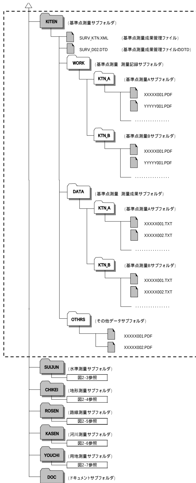
図 2-2 「KITEN」フォルダ内のサブフォルダ構成
