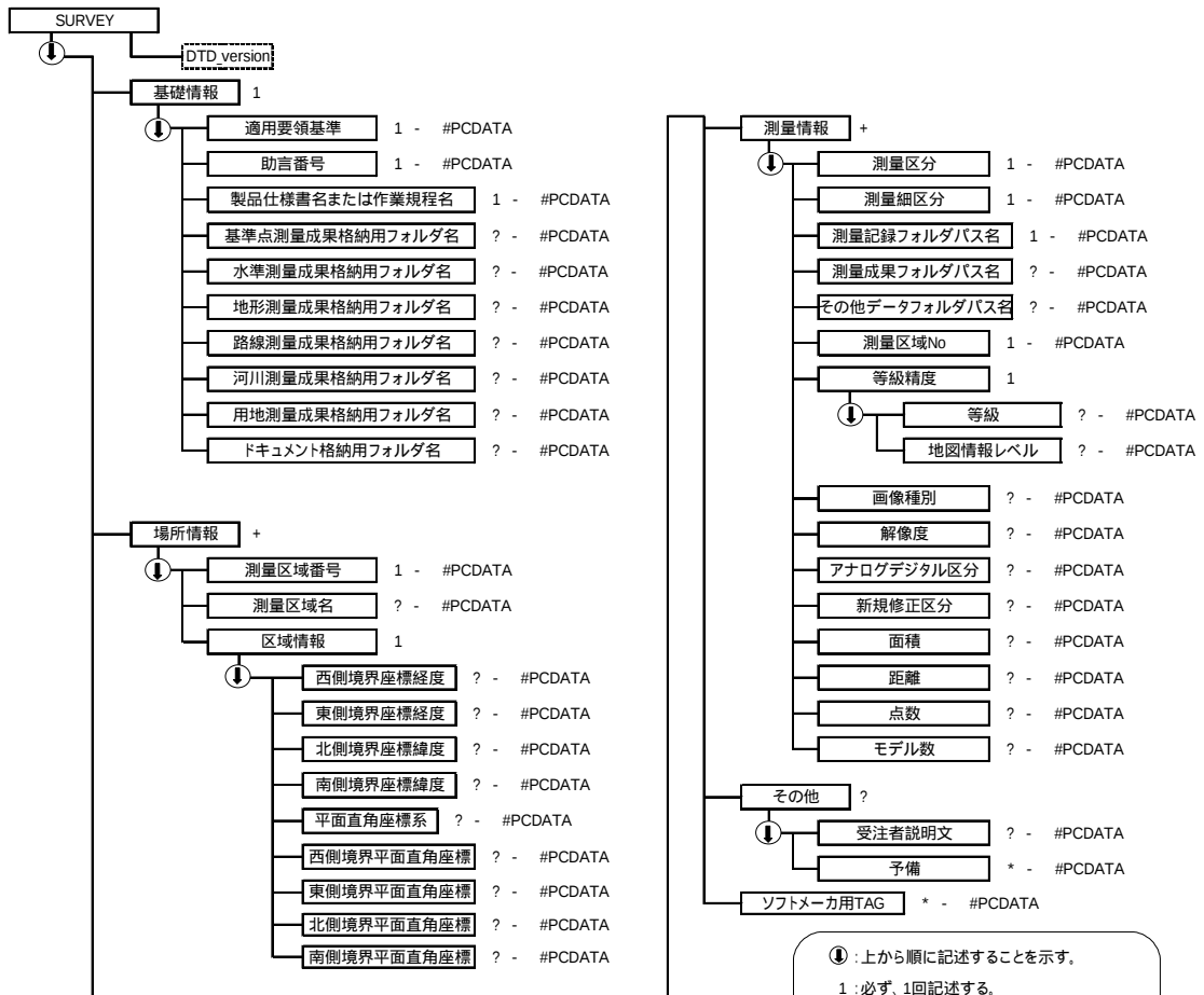
SURVEY02.DTDの構造図
