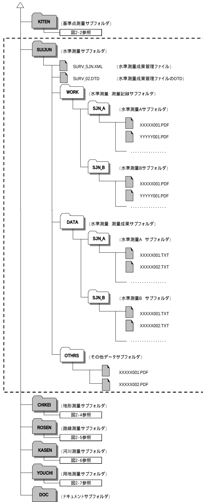
図 2-3 「SUIJUN」フォルダ内のサブフォルダ構成
