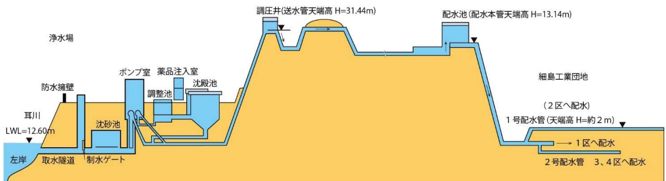
図2 施設概念図
