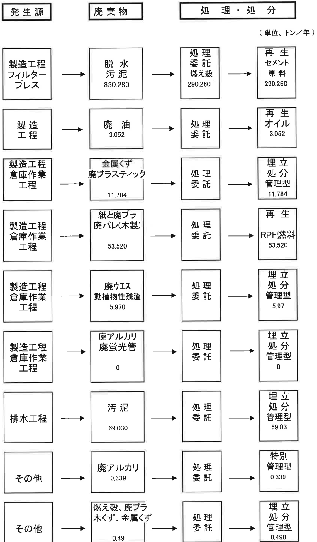
廃棄物処理フロー図 (図一)
