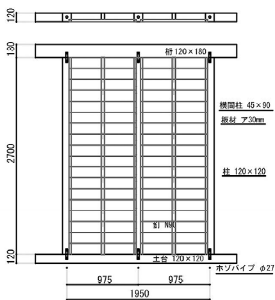
スギ板横貼り工法壁
