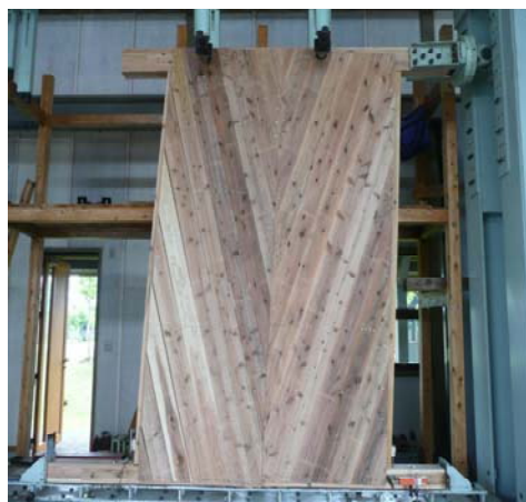
写真2 斜貼り壁試験状況
