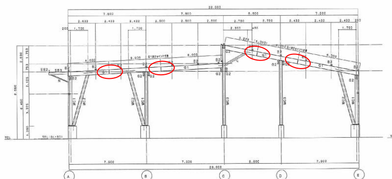
図2 製材工場軸組
