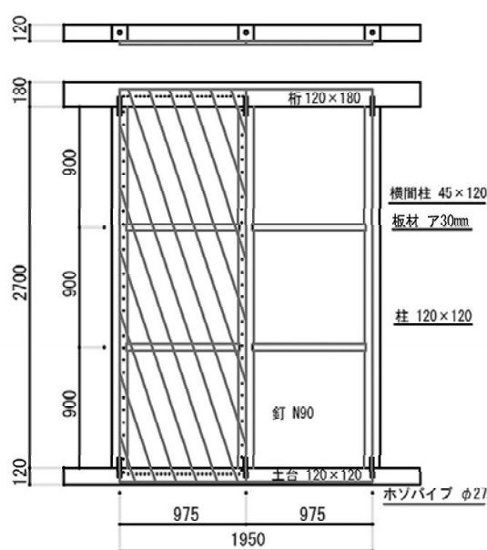
スギ板斜貼り工法壁
