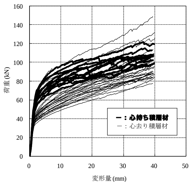
図1 めり込み試験における荷重変形曲線
