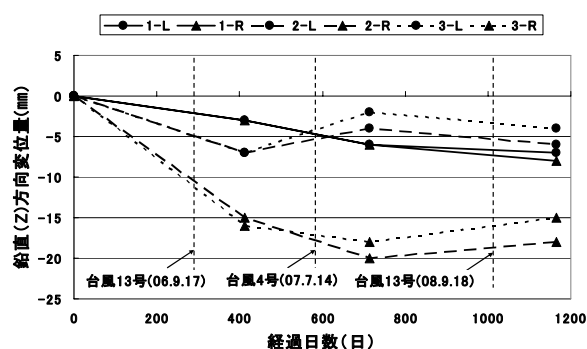
図6 トラスのZ方向変位量と経過日数の関係
