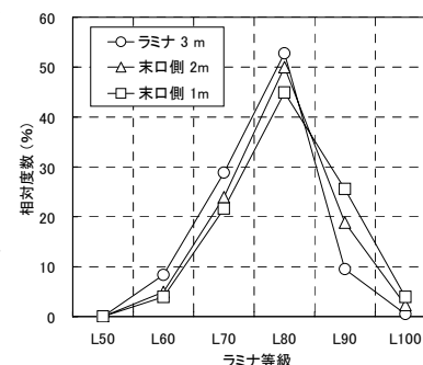
図 2 ラミナの採材位置と等級
