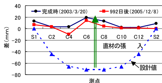
図6 50mキングポストトラスの変位量の推移
