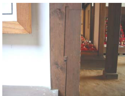
柱の継ぎ手（金輪継ぎ）
