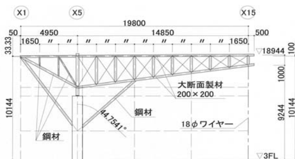
図-2 メイントラス（L3,R3）構造立面
