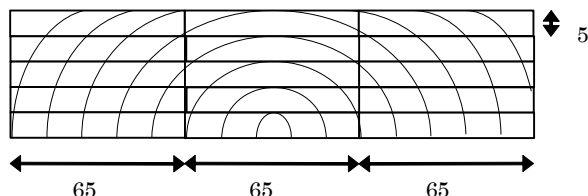
図-1 横断面の含水率測定用試験片の作成方法(単位:mm)
