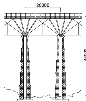
図 3 トレッスル橋のイメージ図
