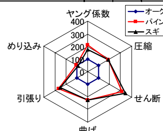
図 2 比ヤング係数・比強度の比較
