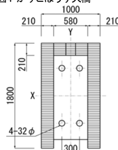
図5 下弦材の断面図
