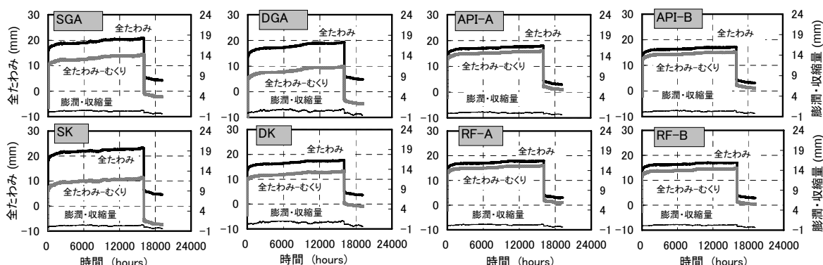
図1 全たわみ(初期たわみ + クリープたわみ)、全たわみーむくり、及び膨潤・収縮量の変動
