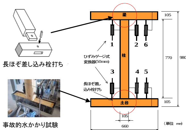
図1 試験体と試験条件
