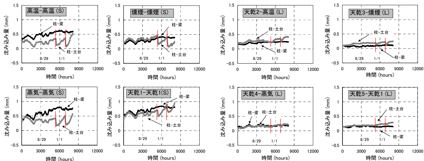
図3 沈み込み量の変動
