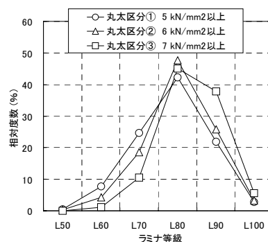
図 1 丸太区分とラミナ等級
