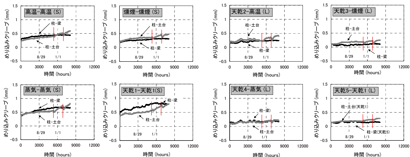
図2 めり込みクリープの変動
