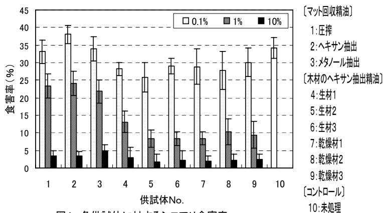
図1 各供試体に対するシロアリ食害率
