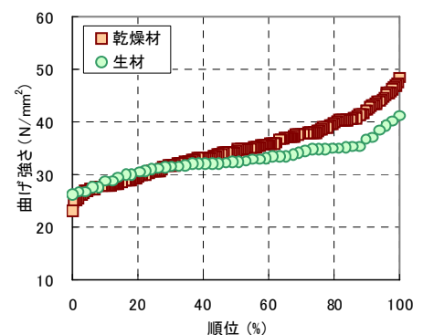
図1 曲げ強さの正規化グラフ
