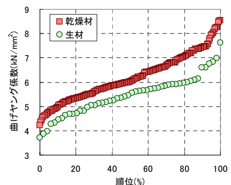
図2 曲げヤング係数の正規化グラフ
