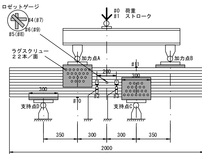
図1 せん断試験方法
