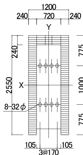
図2 下弦材断面
