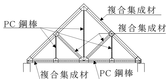
図1 構造モデル
