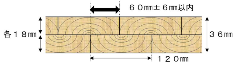
図1 MLTの断面
