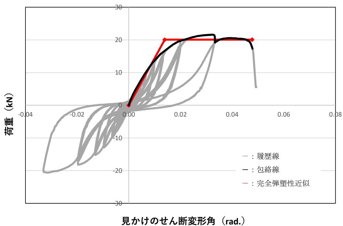
図6 荷重と見かけのせん断変形角の関係（出隅対応型－2 試験体）
