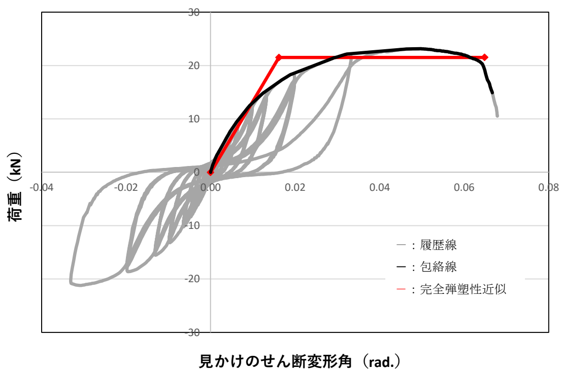
図7 荷重と見かけのせん断変形角の関係（出隅対応型－3 試験体）
