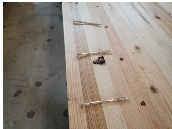
(iv) ビス (MLT－受材接合) の損傷状況
