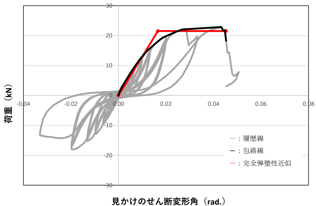
図 5 荷重と見かけのせん断変形角の関係（出隅対応型－1 試験体）
