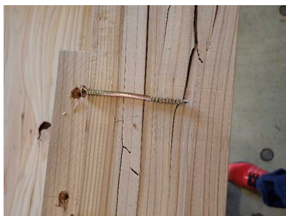
(v) ビス（MLT－受材接合）の損傷状況
