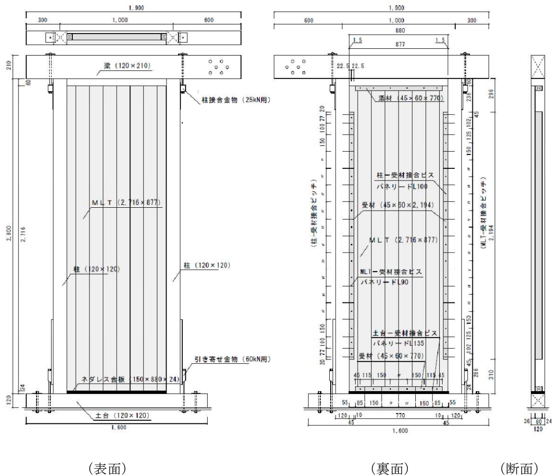
図3 試験体図
