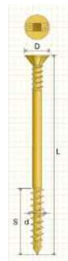
図2 ビス形状
