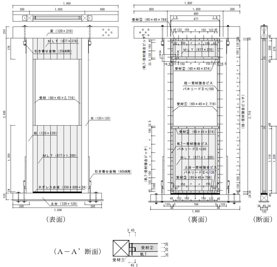
図3 試験体図
