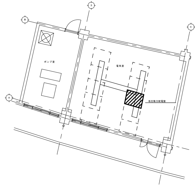
電気室平面詳細図 S=1/50
