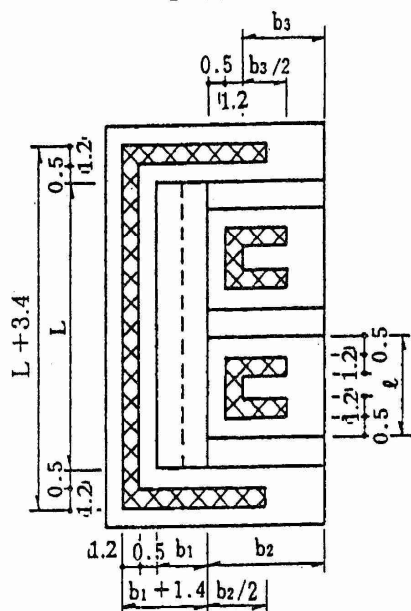
② 平面図
