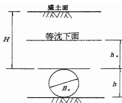
図1 寸法表示 (突出形)
