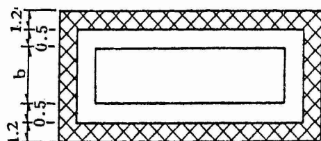
① 平面図
