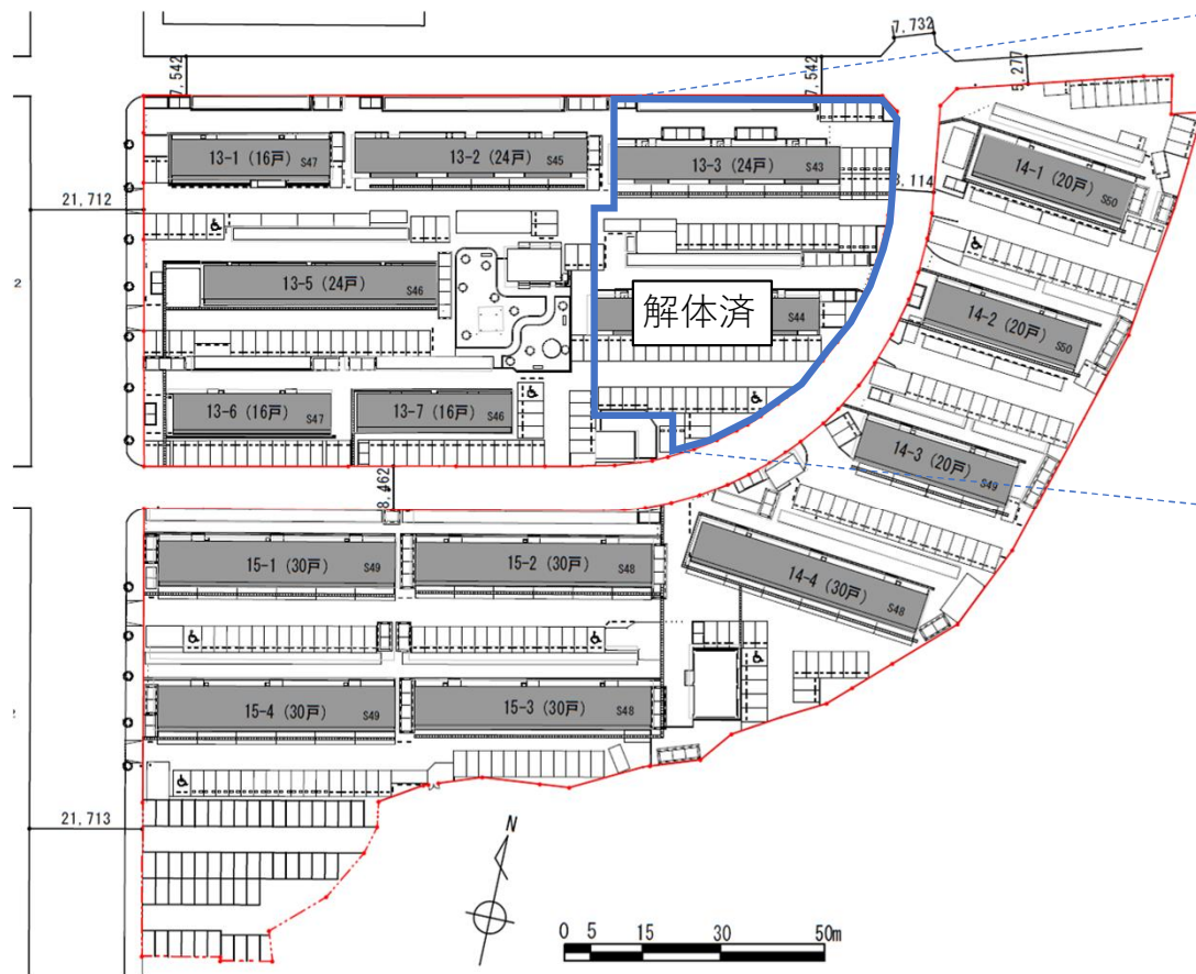
現況配置図
