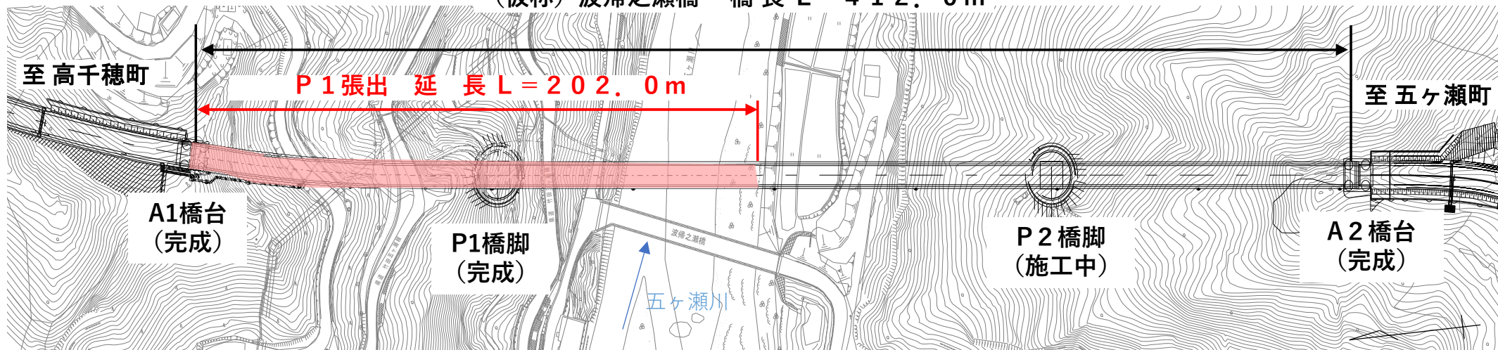
平面図
