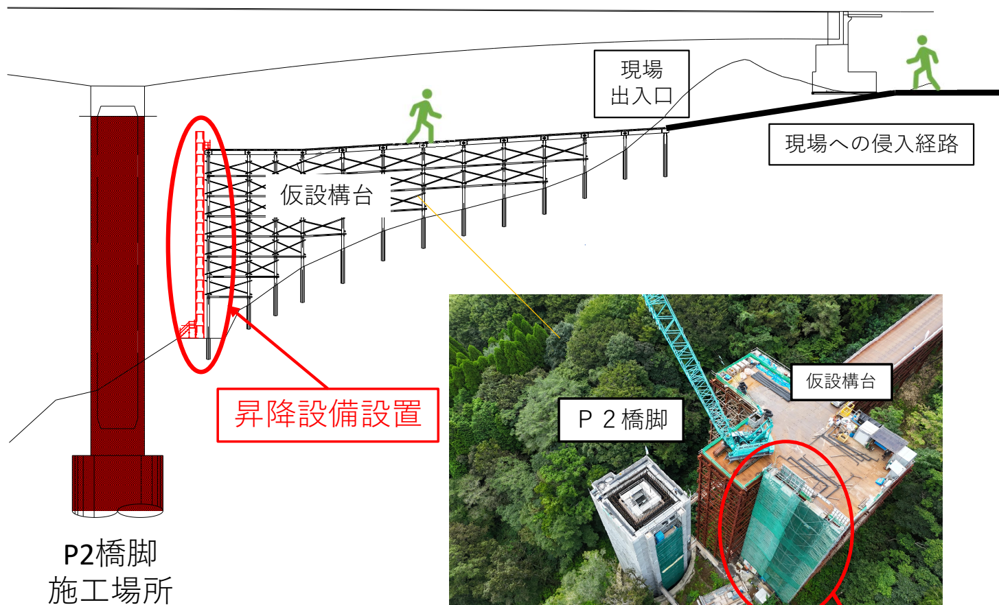
側面図
