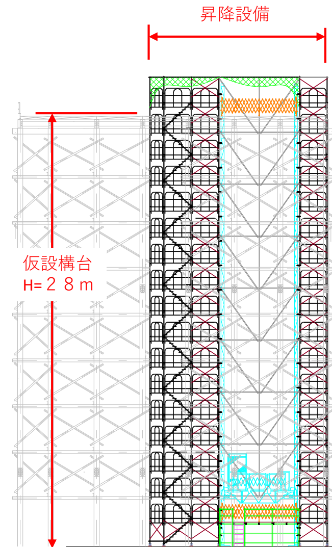
正面図
