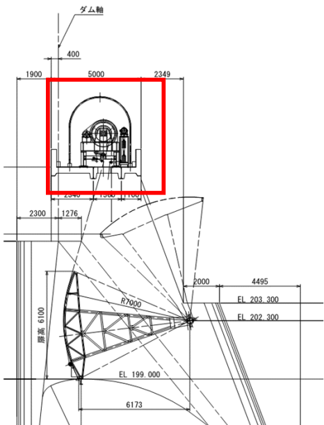
断面図
