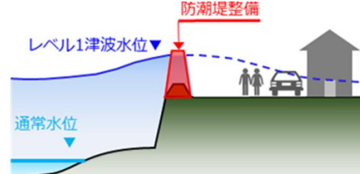
海岸防潮堤の地震津波対策
