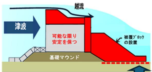
基礎部分の強化により倒壊を防ぐ
