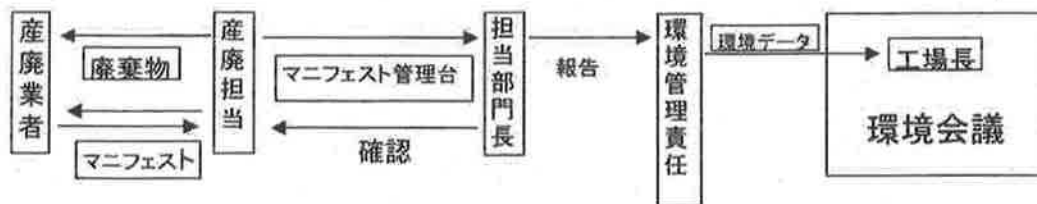
(管理体制図)
