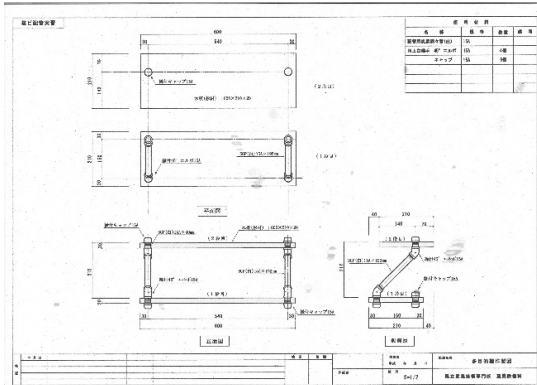
制作棚図面
